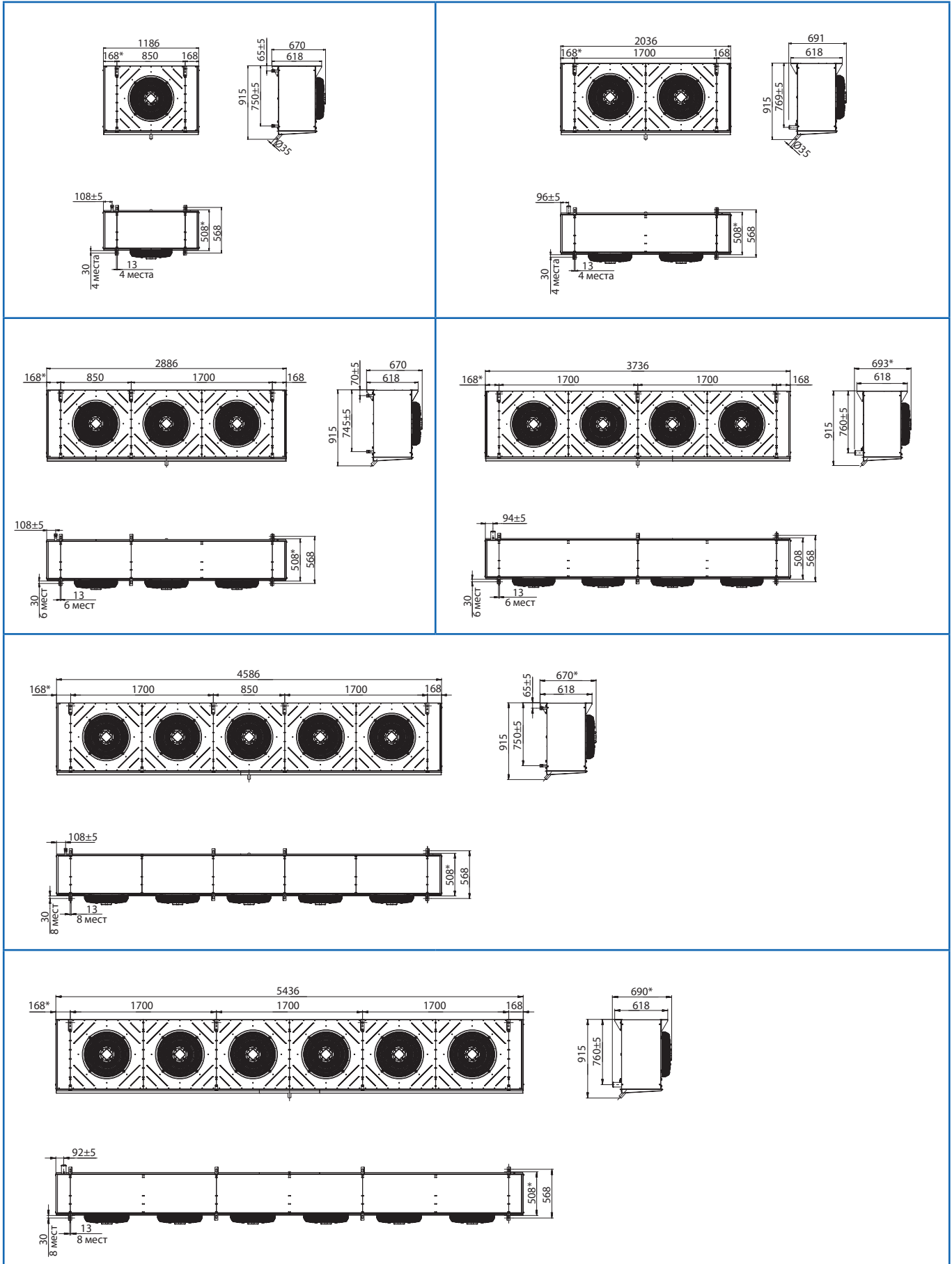
Габаритные и присоединительные размеры UCR.500
