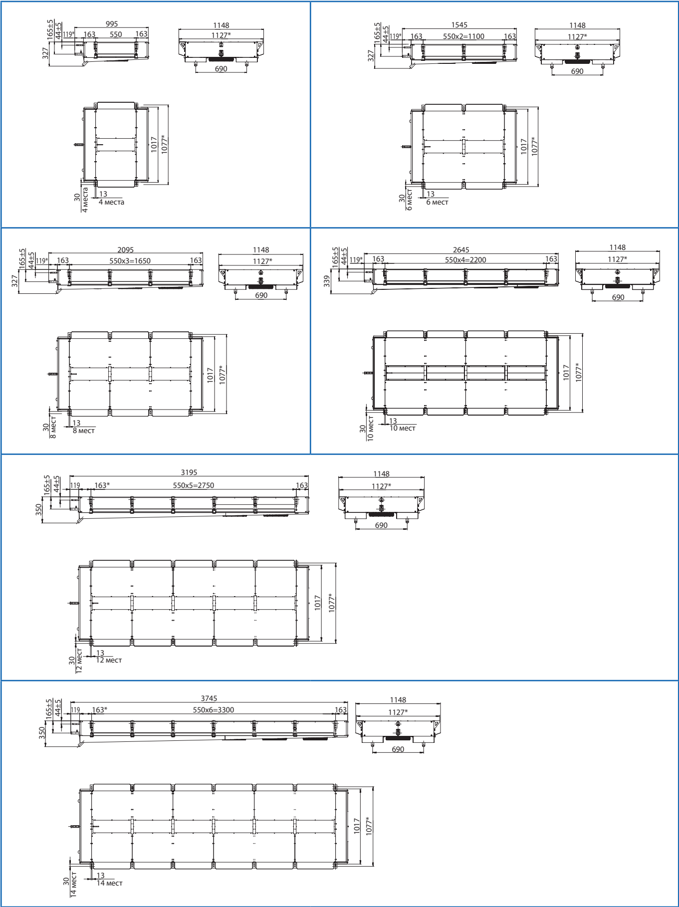
Габаритные и присоединительные размеры UDR.300
