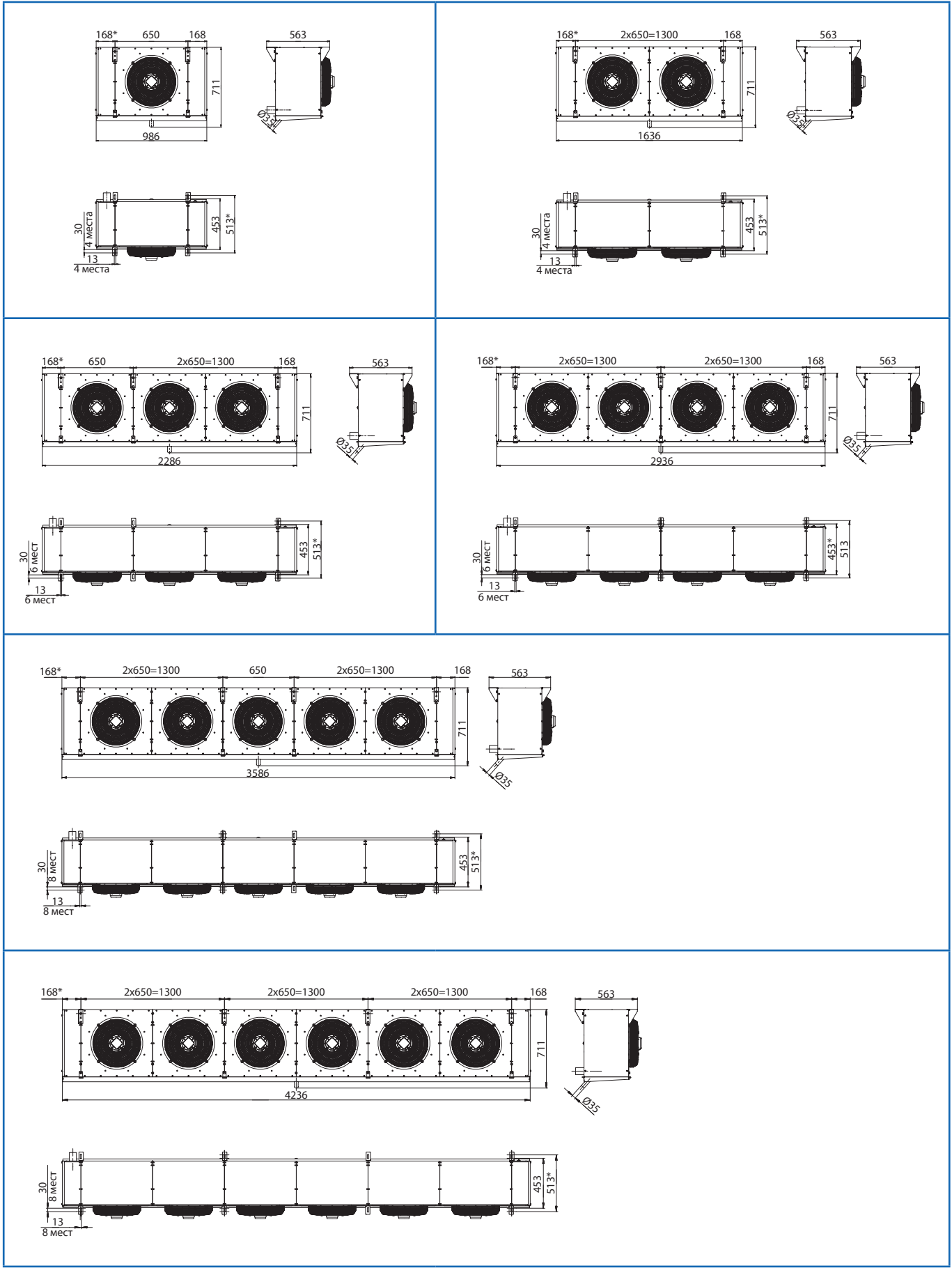
Габаритные и присоединительные размеры UCR.400
