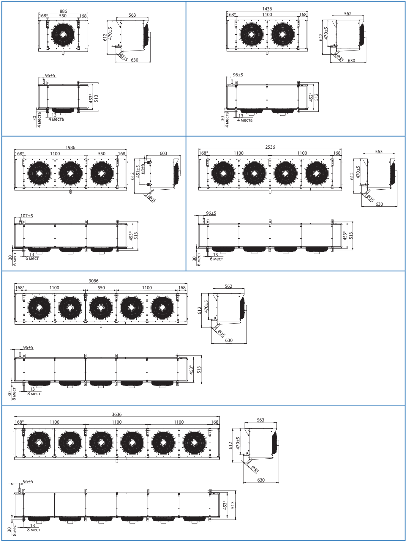
Габаритные и присоединительные размеры UCR.350
