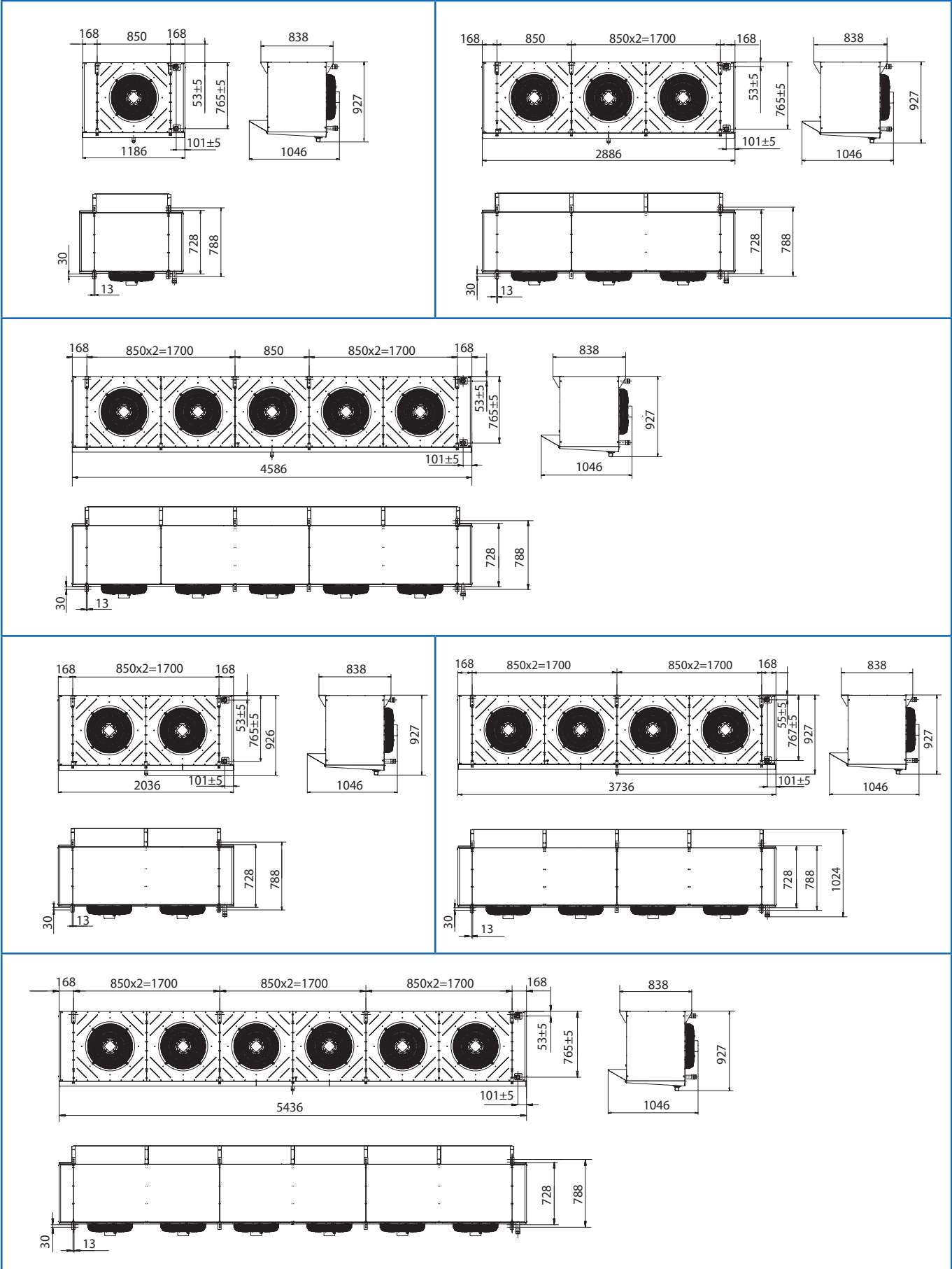
Габаритные и присоединительные размеры UCRA
