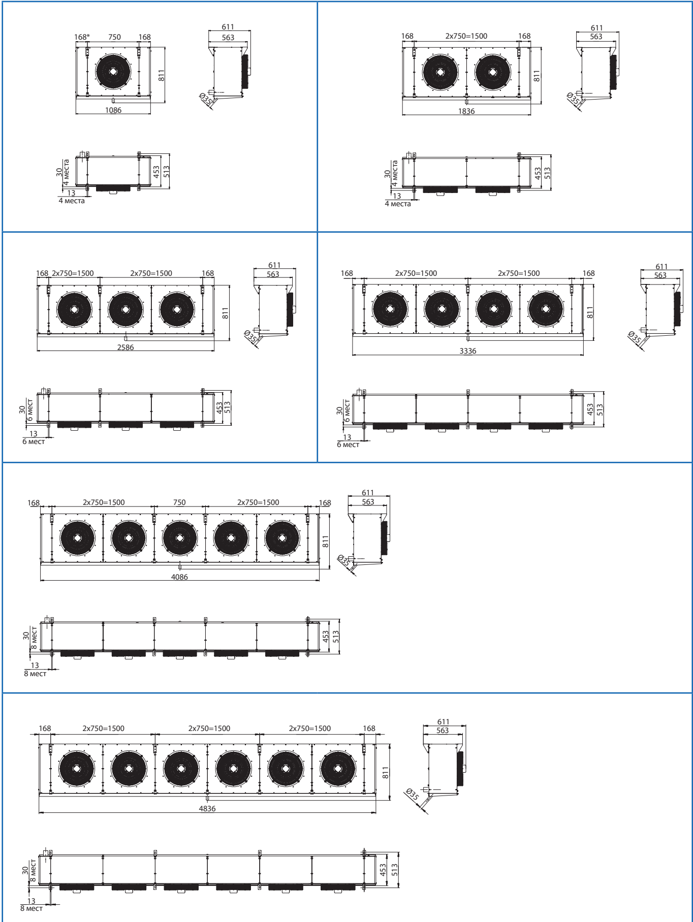
Габаритные и присоединительные размеры UCR.450
